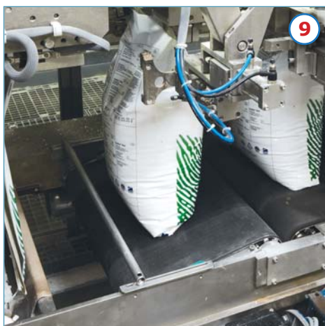
9 Nastro sbattitore per compattamento prodotto all'interno del sacco - Shaking belt for product squaring inside the bag - Tapis mélangeur pour compactage produit à l'intérieur du sac
